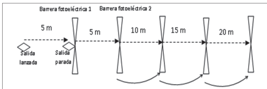
FIGURA 3. Esquema distribución barreras fotoeléctricas
